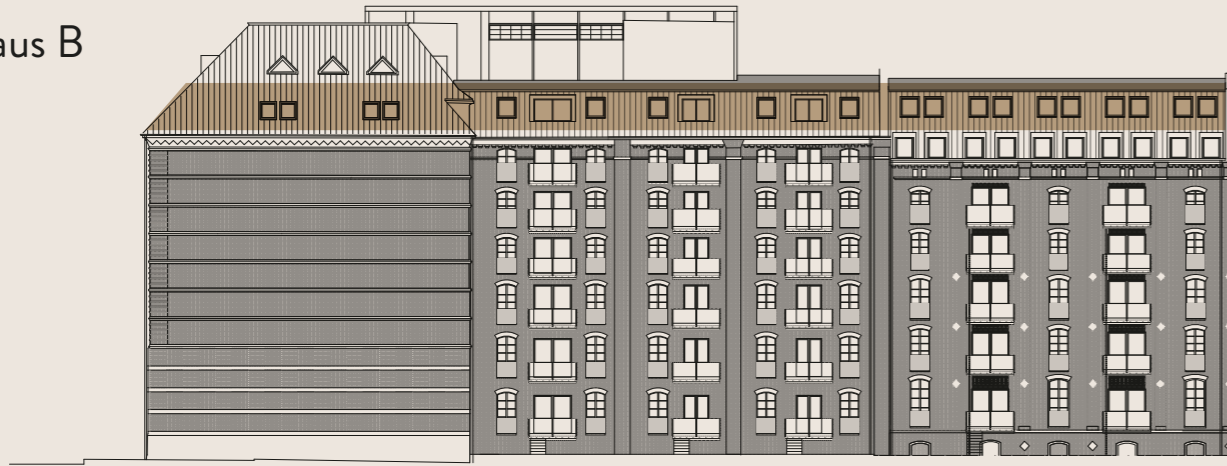
Ansicht Ost
